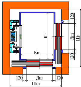
Проходная кабина на 90 градусов для электрического лифта МиниБМП
